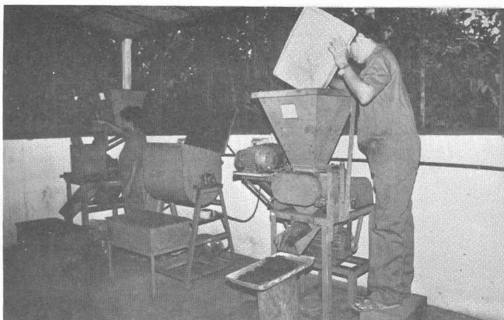
Fig. 2. Planta piloto utilizada na fabricação do briquete.
